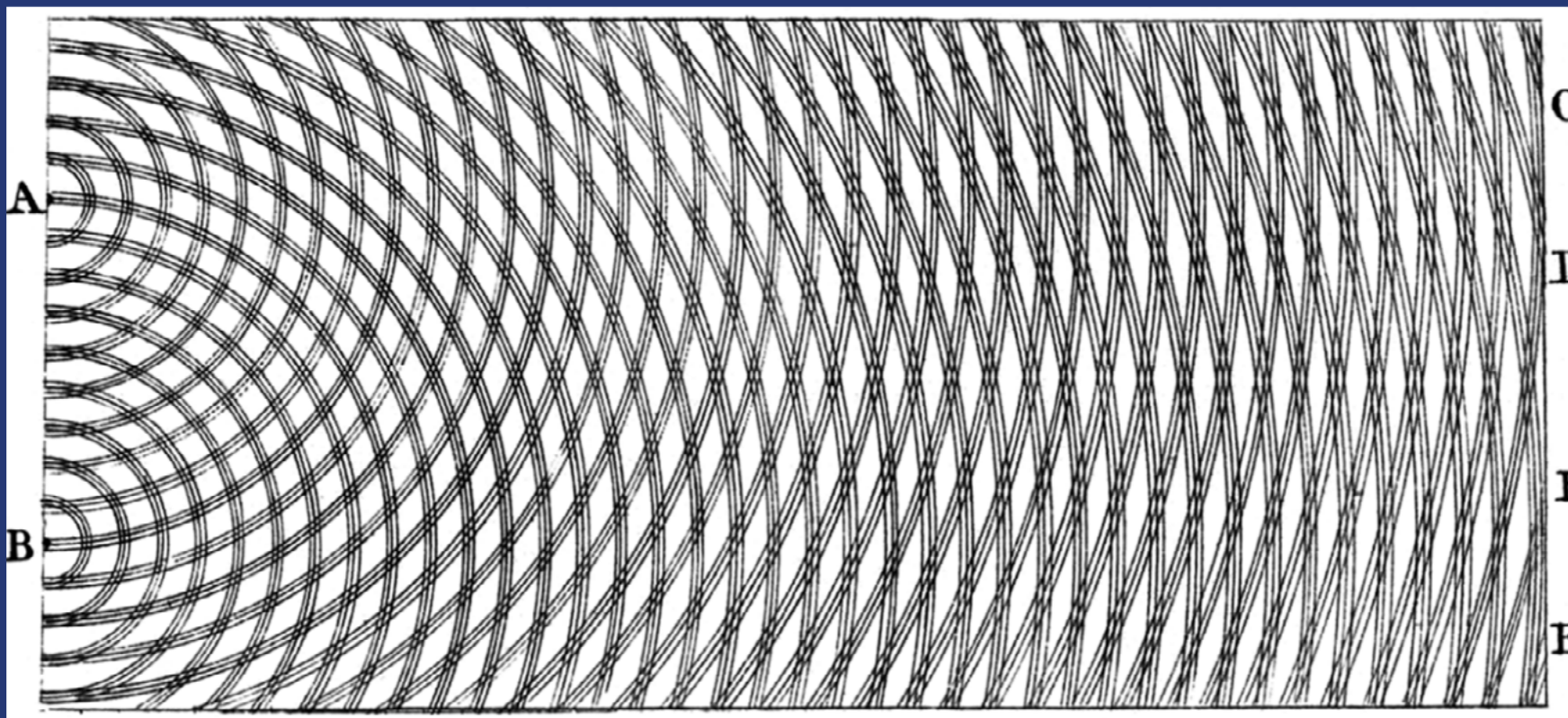
Desenul lui Thomas Young ce prezintă interferența generată de două unde coerente prezentată Societății Regale în 1803. Cele două surse-fantă sunt poziționate în punctele A și B, iar diferite faze ale interferenței sunt figurate prin punctele C, D, E și F.
